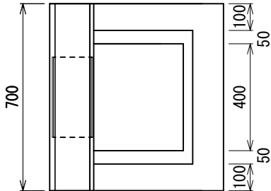
標準型縁塊 FS-A 131kg
