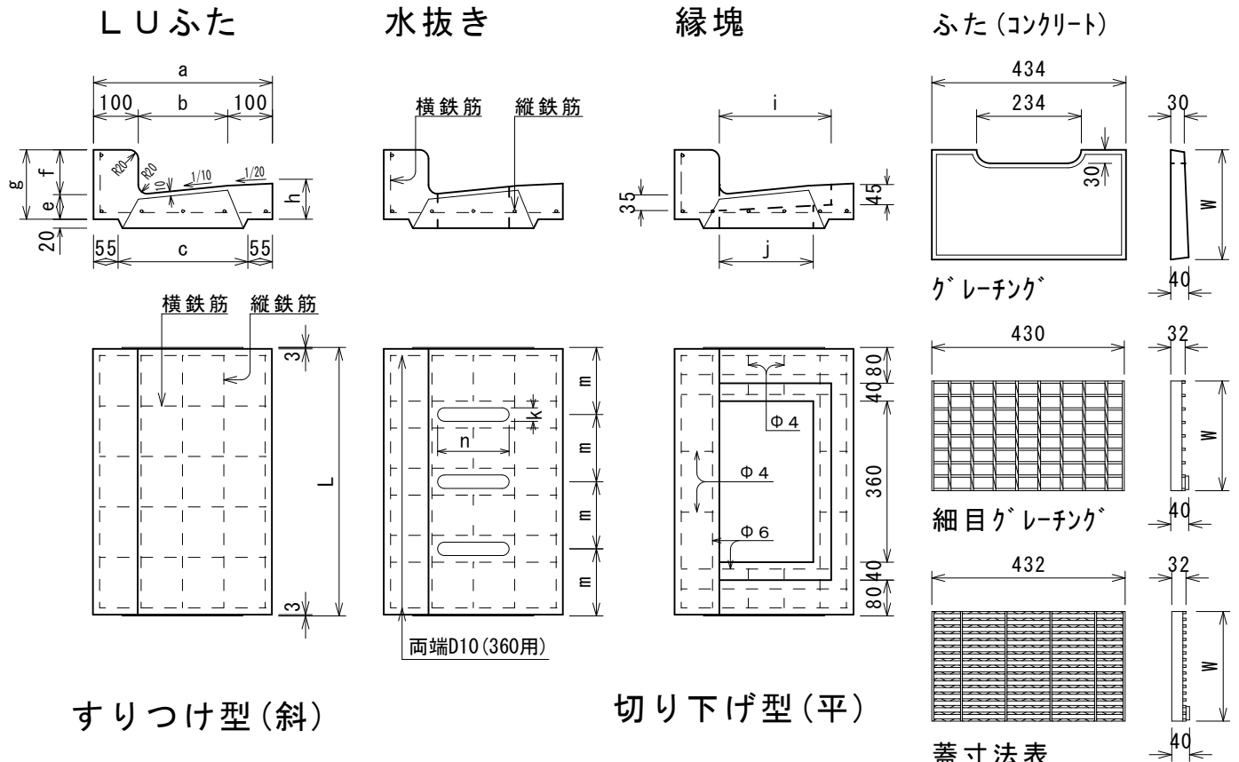
蓋寸法表
