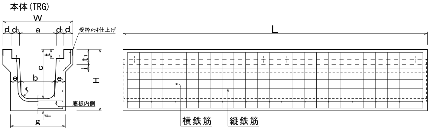
寸法及び配筋表
