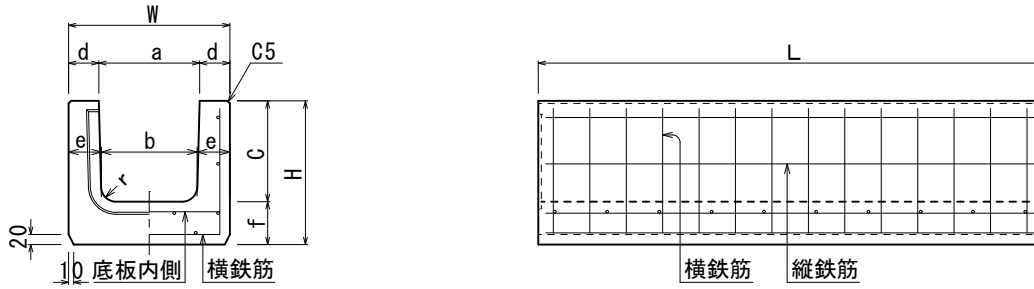
寸法及び配筋表
