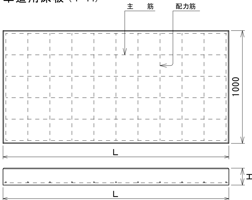
寸法及び配筋表
