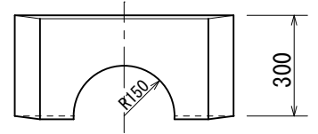
1号 有孔下 99kg
