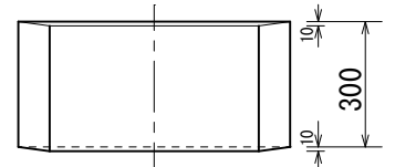
2号 有孔上 99kg
