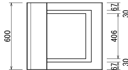
寸法表
