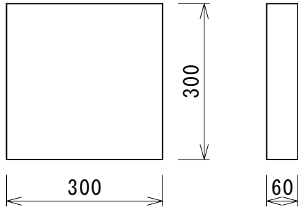
平板 13kg
