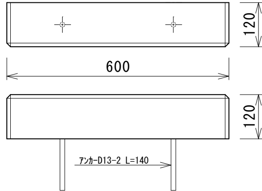
車止め(地先アンカー付) 21kg
