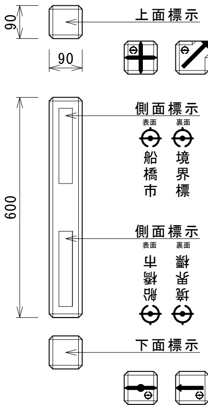
境界杭
