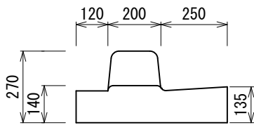
すりつけ型 FT-BF 463kg
