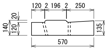
切り下げ型 FD-BF 358kg
