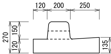
水抜き型 FS-BF 471kg
