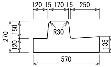
水抜き型 FS-BF 471kg
