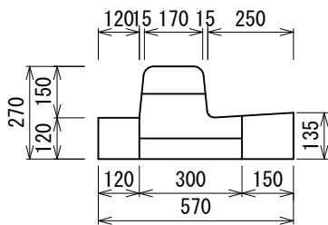
標準型縁塊 FS-BF 122kg
