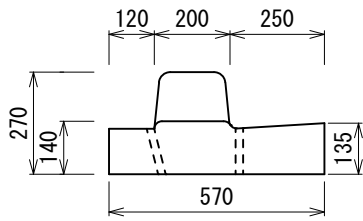
すりつけ型 FT-BF 455kg
