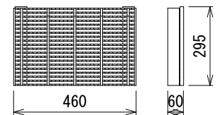
細目スベリ止めグレーチング 15.9kg
