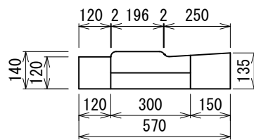
切り下げ型縁塊 FD-BF 81kg
