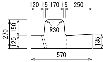
標準型 FS-BF 475kg
