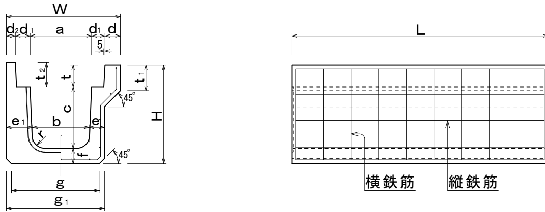
寸法及び配筋表
