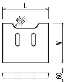
ふた (155・205A) ( )内乗入用
