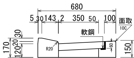
車乗入縁塊 (両面) 155 86kg
