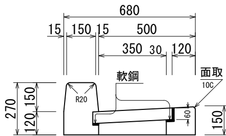
車乗入縁塊 (両面) 155 86kg
