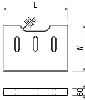
グレーチング
