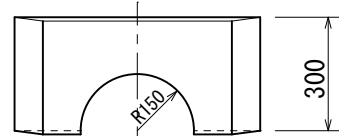
1号 有孔下 99kg
