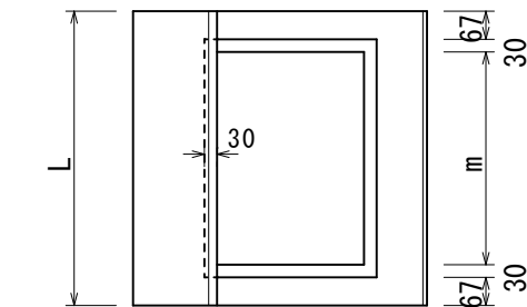
ふた (155・205A) ( )内乗入用
