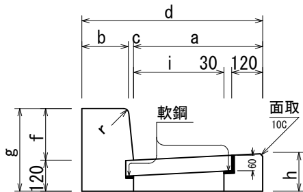
縁塊 (155R面取り) 113kg
