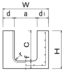
寸法及び配筋表
