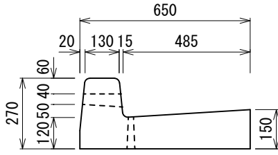
I 型 標準型 FS-A 514kg
