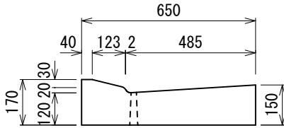
切り下げ型 MD-A1 444kg
