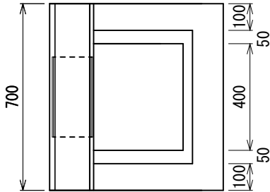
標準型縁塊 FS-A 130kg
