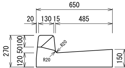
切り下げ型 FD-A 433kg
