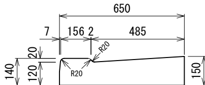
切り下げ型 FD-A 433kg
