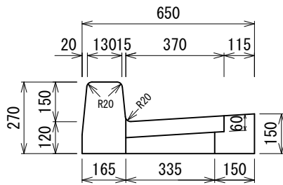
標準型縁塊 FS-A 136kg
