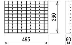
グレーチング T-25 15.2kg
