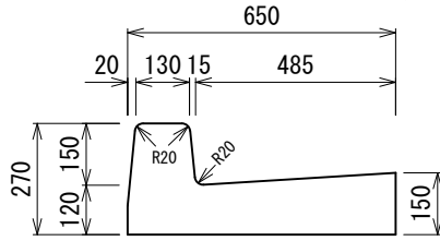
水抜き型 FS-A 517kg
