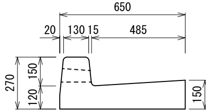
すりつけ型 FT-A 509(142kg)
