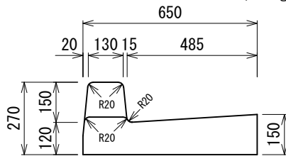
すりつけ型 FT-A 1 512(145kg)
