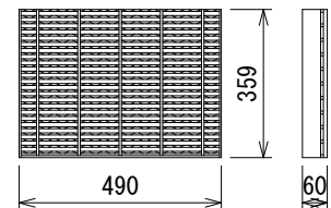
細目スベリ止めグレーチング T-25 20.4kg
