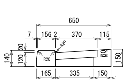
切り下げ型縁塊 FD-A 104kg
