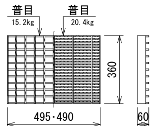
グレーチング
