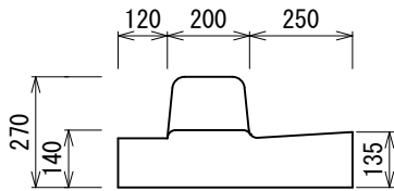
すりつけ型 FT-BF 460kg
