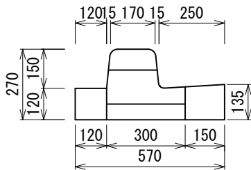
標準型縁塊 FS-BF 125kg
