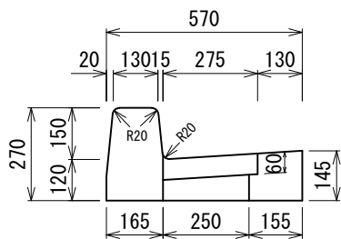
標準型縁塊 FS-A 129kg
