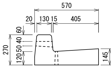
I 型 標準型 FS-A 456kg
