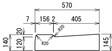
標準型縁塊 FS-A 129kg
