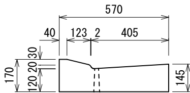
切り下げ型 MD-A1 387kg
