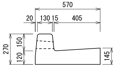
すりつけ型 FT-A 451 (125kg)
