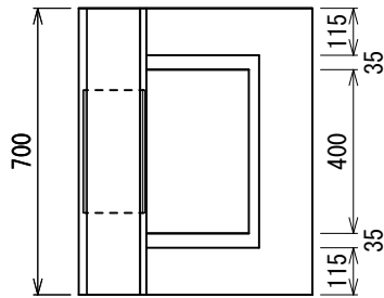
標準型縁塊 FS-A 123kg
