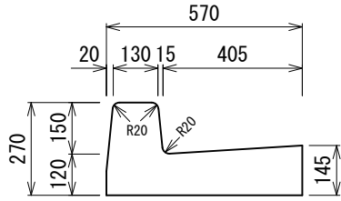
水抜き型 FS-A 459kg
