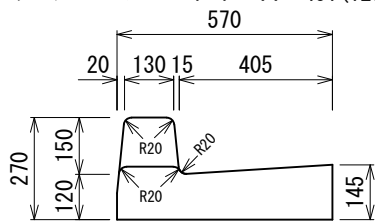
すりつけ型 FT-A1 455 (129kg)
