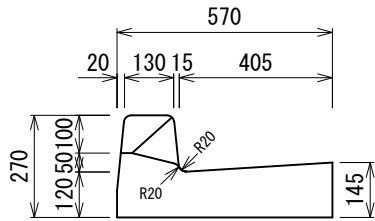
切り下げ型 FD-A 376kg
