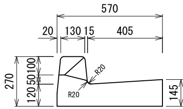
すりつけ型 FT-A1 127kg
