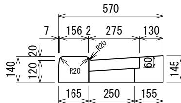
切り下げ型縁塊 FD-A 97kg
