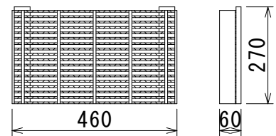
細目グレーチング T-25 14.1 kg
