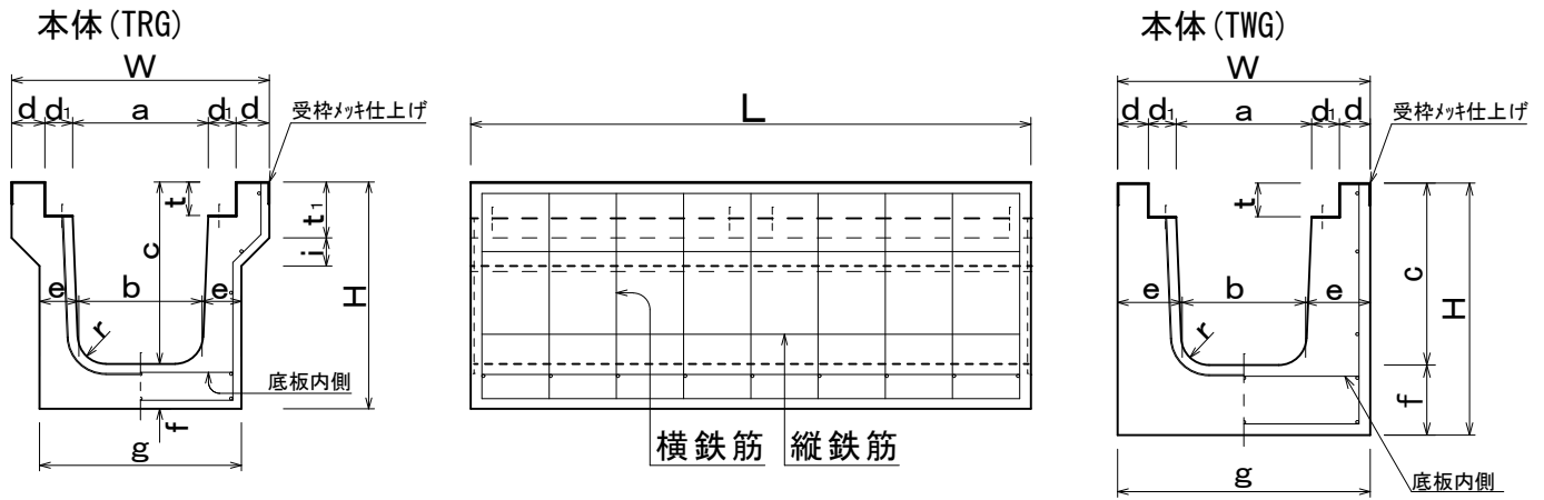
寸法及び配筋表
