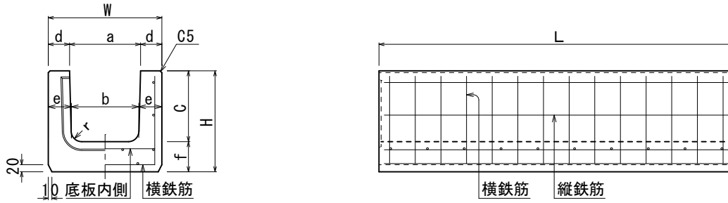
底板内側 寸法及び配筋表
