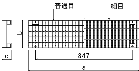
グレーチング寸法表
